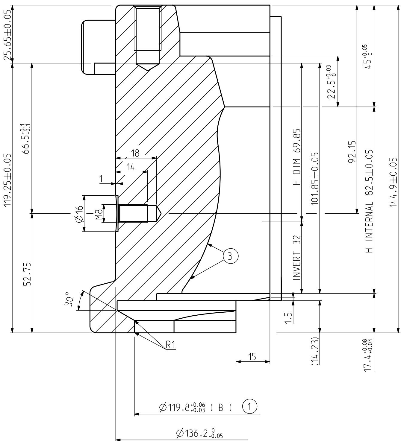
DELIVELLAZIONE AL CENTRO DI -0.08±0.01 SULLA META' FEMMINA HOLLOW MILL -0.08±0.01 FEMALE HALF
