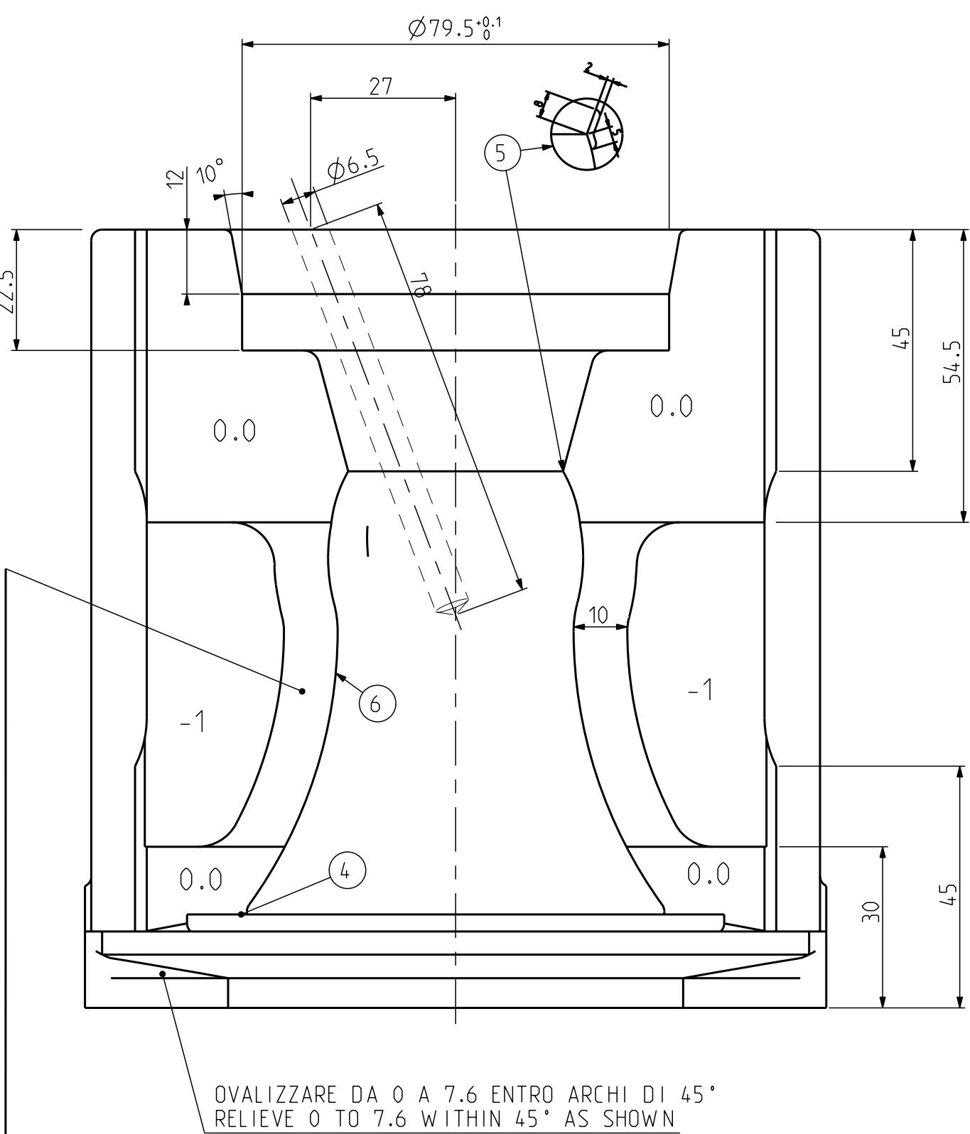
DELIVELLAZIONE AL CENTRO DI -0.08±0.01 SULLA META' FEMMINA HOLLOW MILL -0.08±0.01 FEMALE HALF
